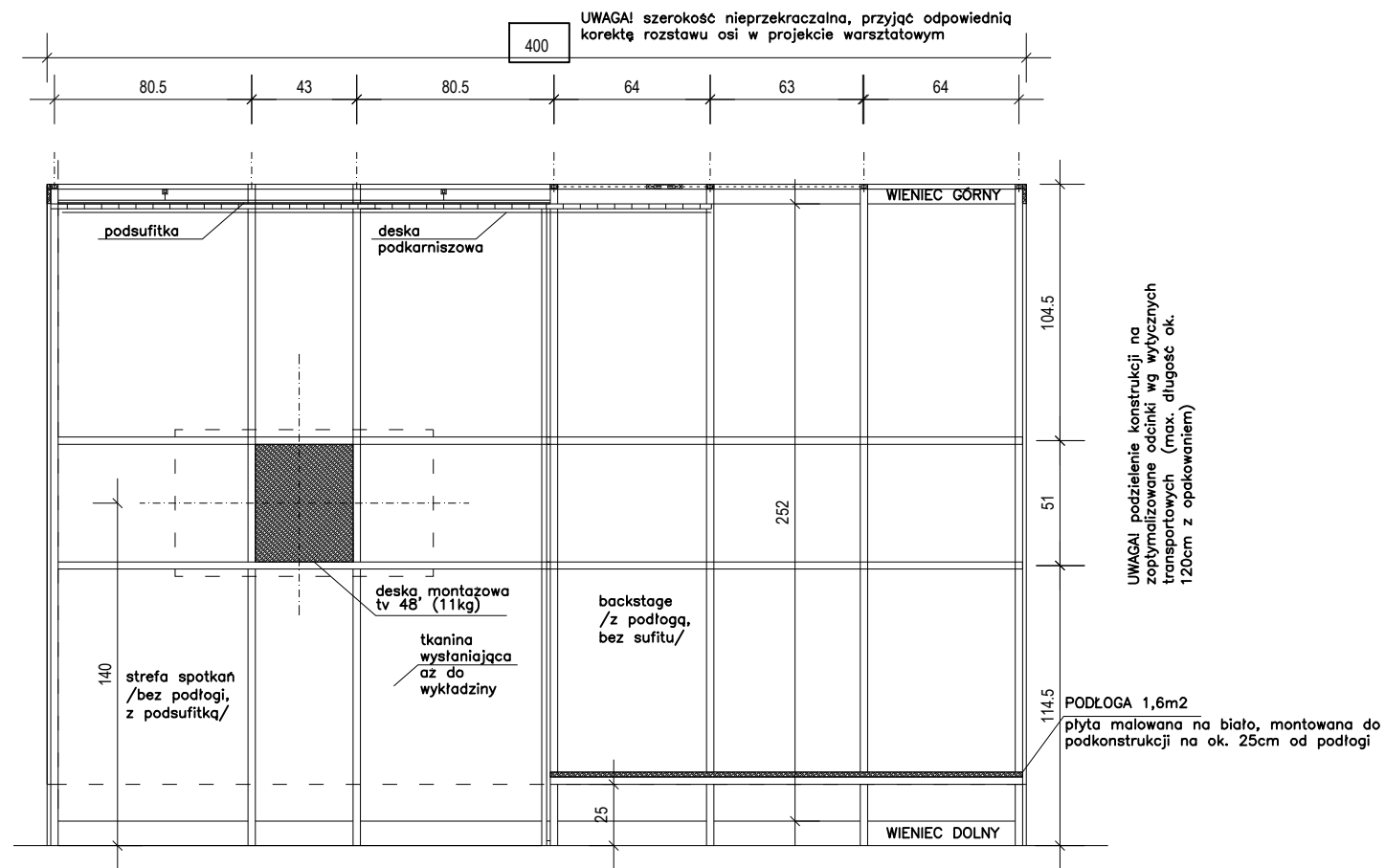
ŚCIANA TYLNA widok od środka formy
